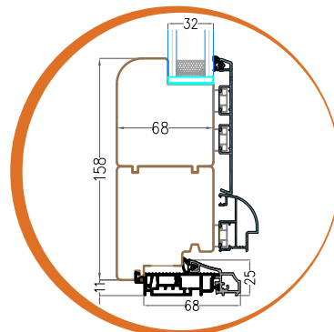
nodo inferiore PORTAFINESTRA "EASY BOLD" Soglia in alluminio H 25 mm con taglio termico
