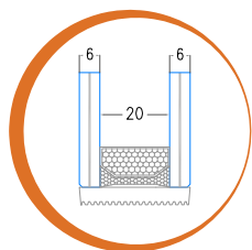
Vetro di serie montato sugli infissi "EASY-BOLD" 33.1be+20argon+33.1 Top1 canalina calda
